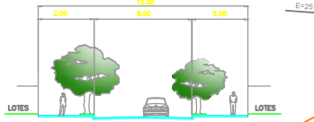
DETALHE DAS RUAS 4, 26 e 31 LARGURA 12,00 metros SEM ESCALA
