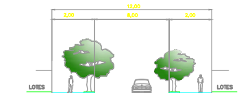
DETALHE DAS RUAS LARGURA 12,00 metros SEM ESCALA
